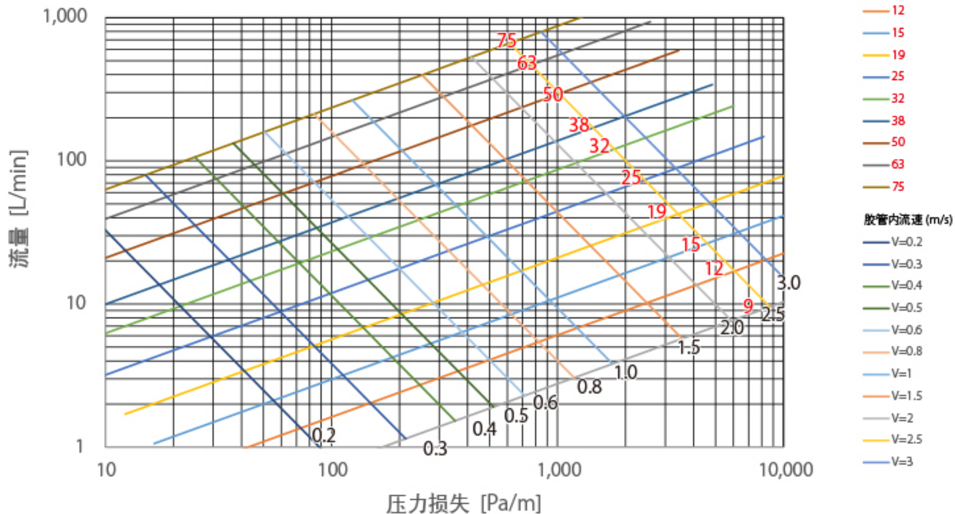
流量线图 (水温25℃)
