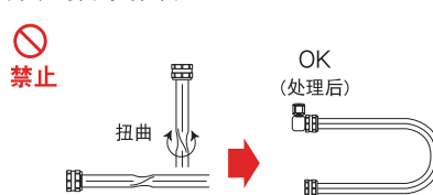
例2) 弯曲时的扭曲
